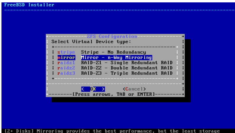
図2.20 ZFS プールタイプ
