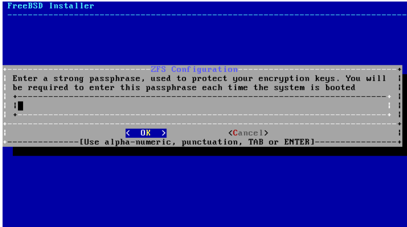
図2.24 ディスク暗号化パスワード
