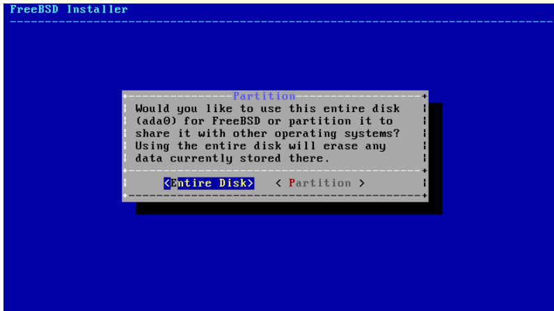
図2.14 Entire Disk または Partition の選択
